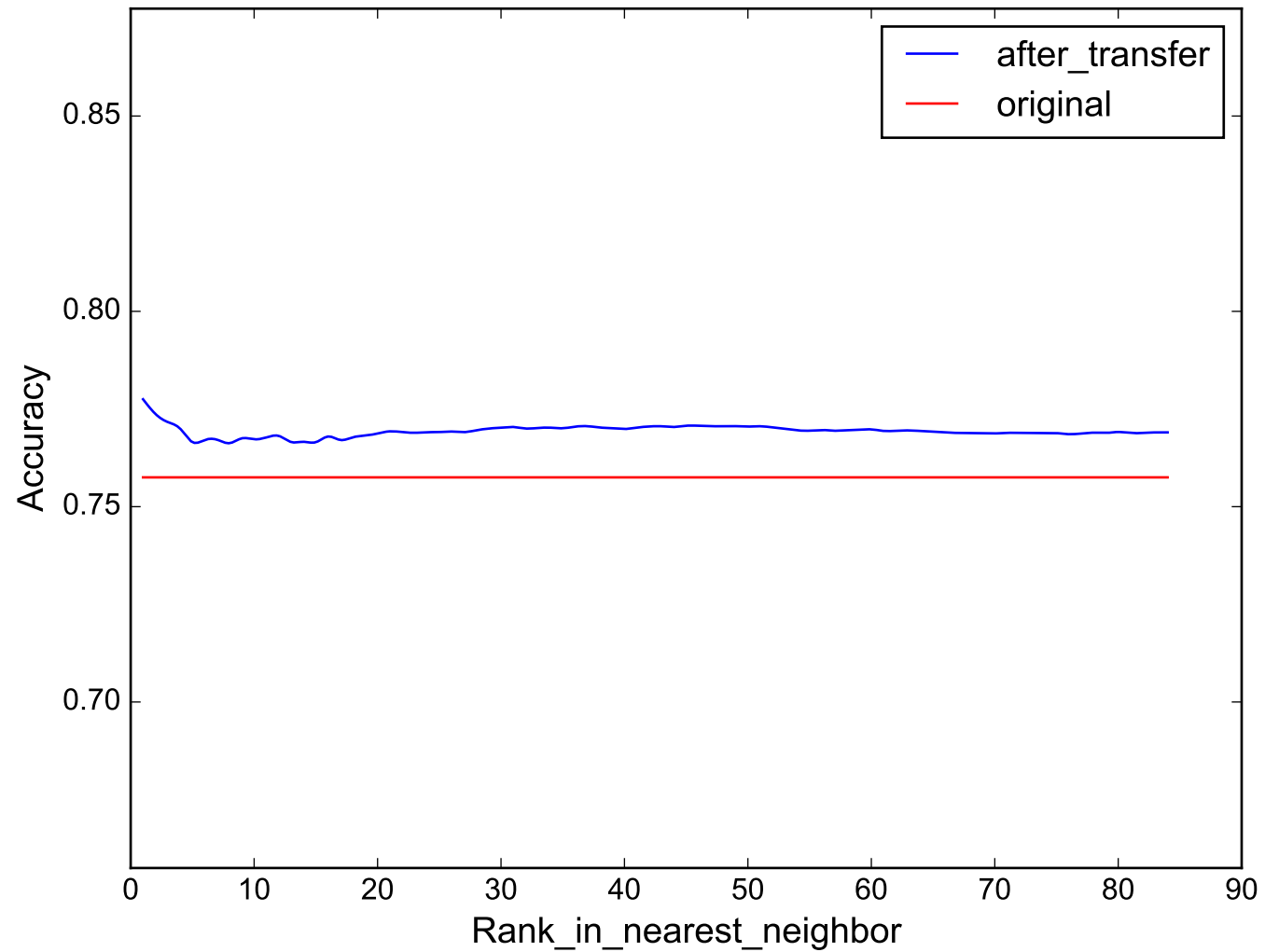
DistalPhalanxTW
