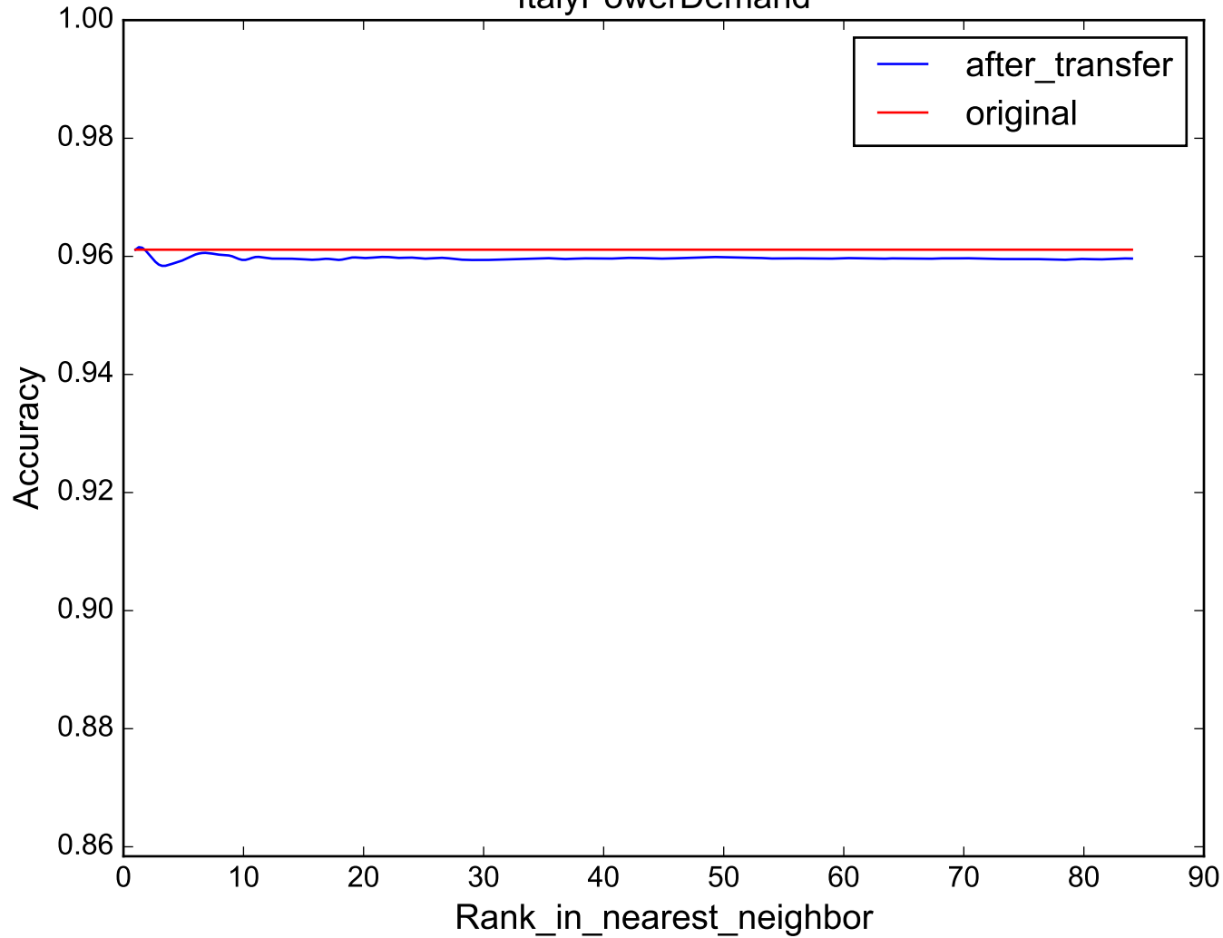
ItalyPowerDemand
