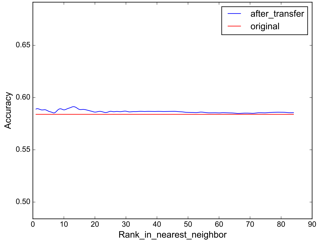
MiddlePhalanxTW
