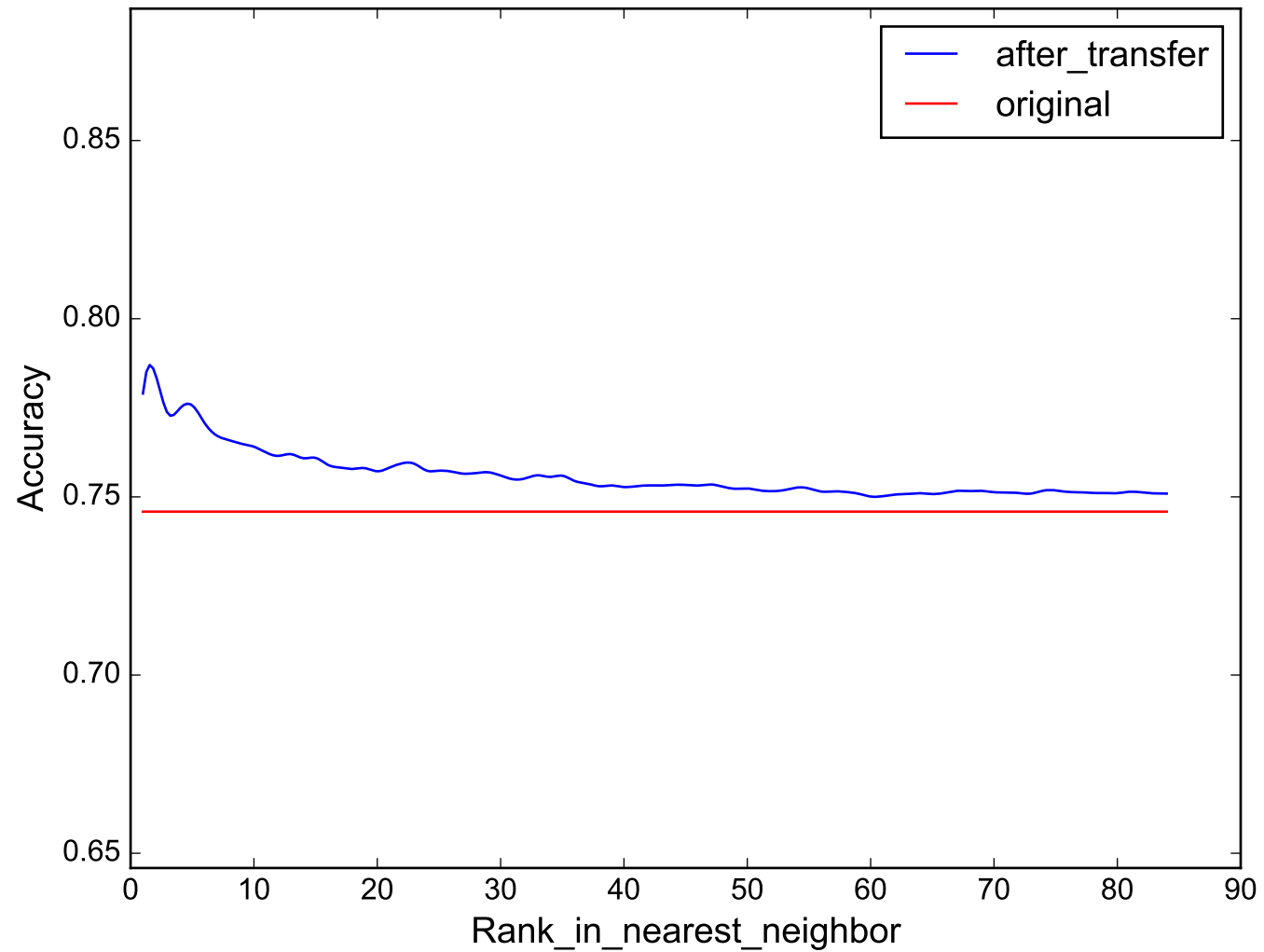
WormsTwoClass
