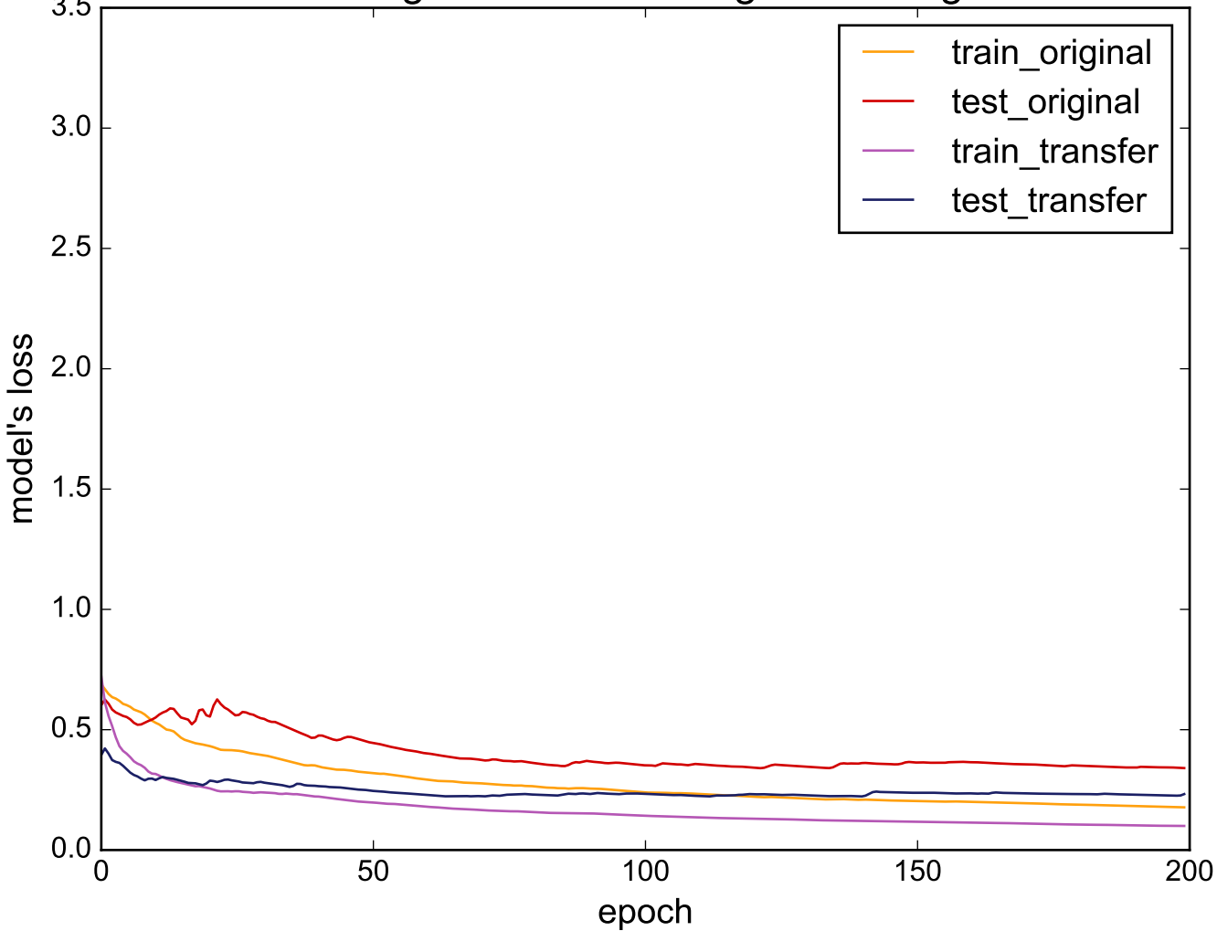
Source: ToeSegmentation2 - Target: ToeSegmentation1
