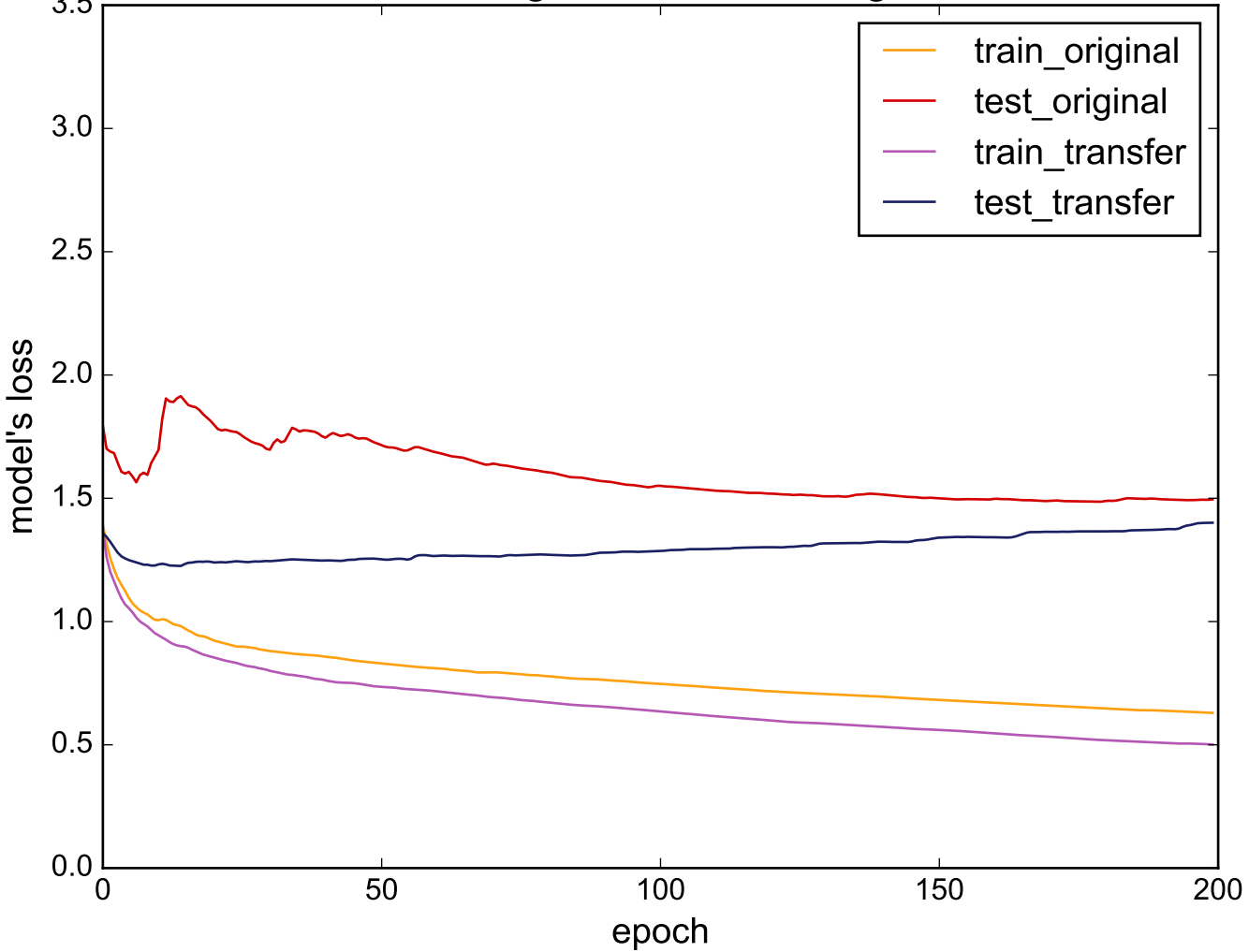
Source: ToeSegmentation2 - Target: Worms
