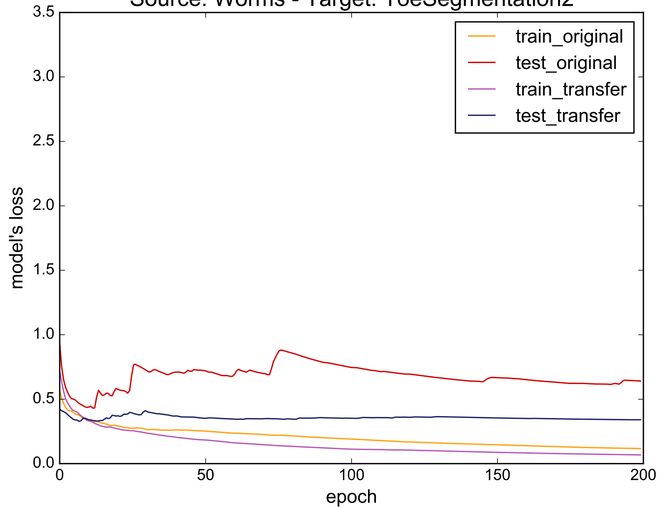
Source: Worms - Target: ToeSegmentation2
