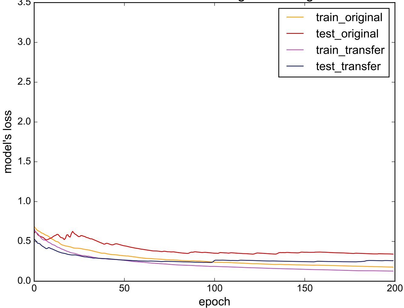
Source: WormsTwoClass - Target: ToeSegmentation1
